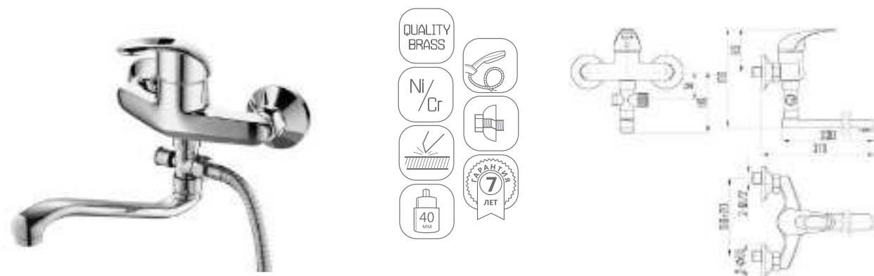
DVL0321-04 Смеситель для ванны с поворотным изливом и наружным кнопочным дивертором, хром
